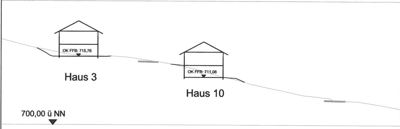
Schnitt 2 - 2; M 1 : 500
