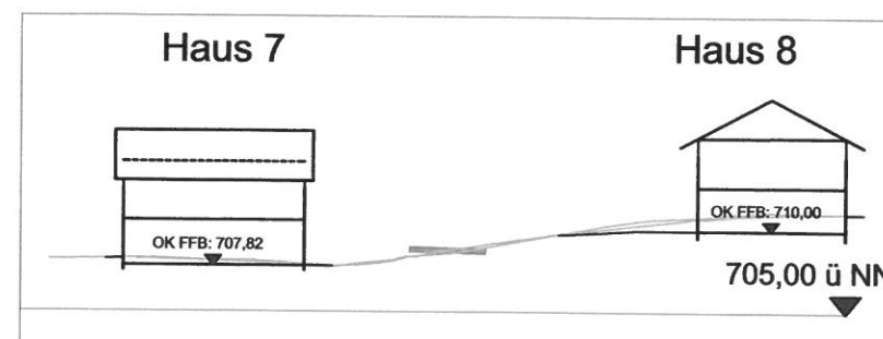
Schnitt 6 - 6; M 1 : 500
