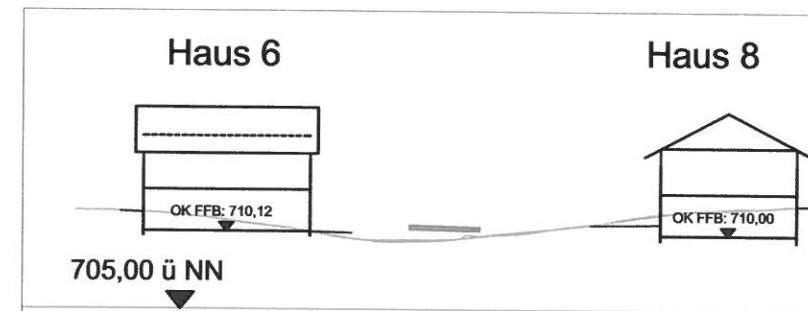
Schnitt 5 - 5; M 1 : 500
