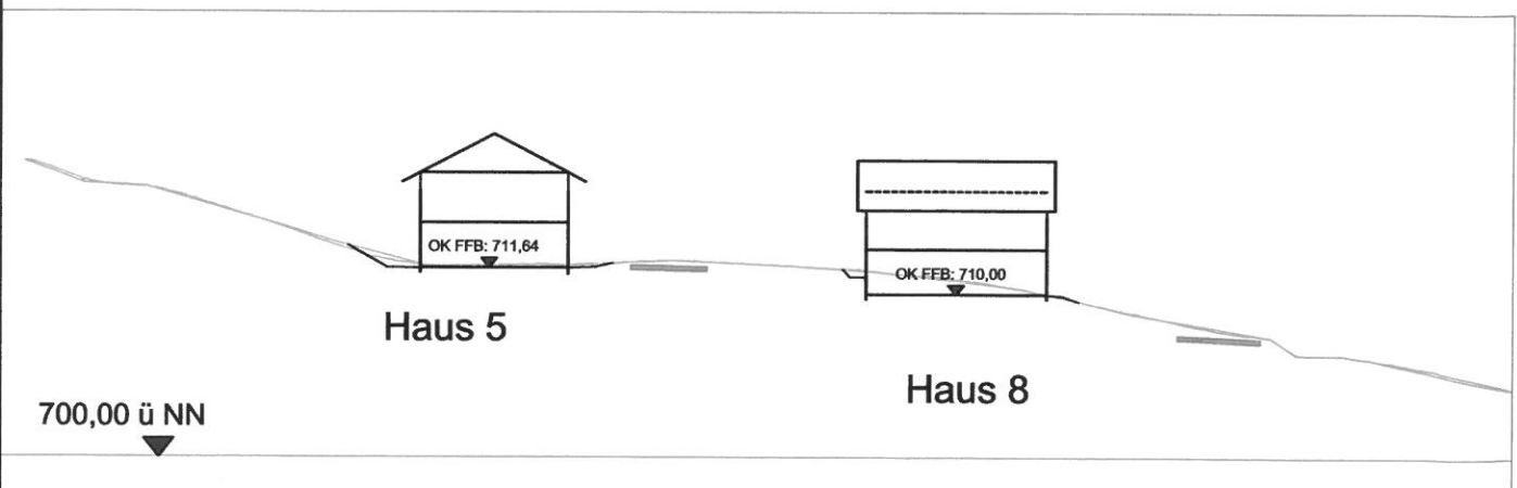
Schnitt 4 - 4; M 1 : 500
