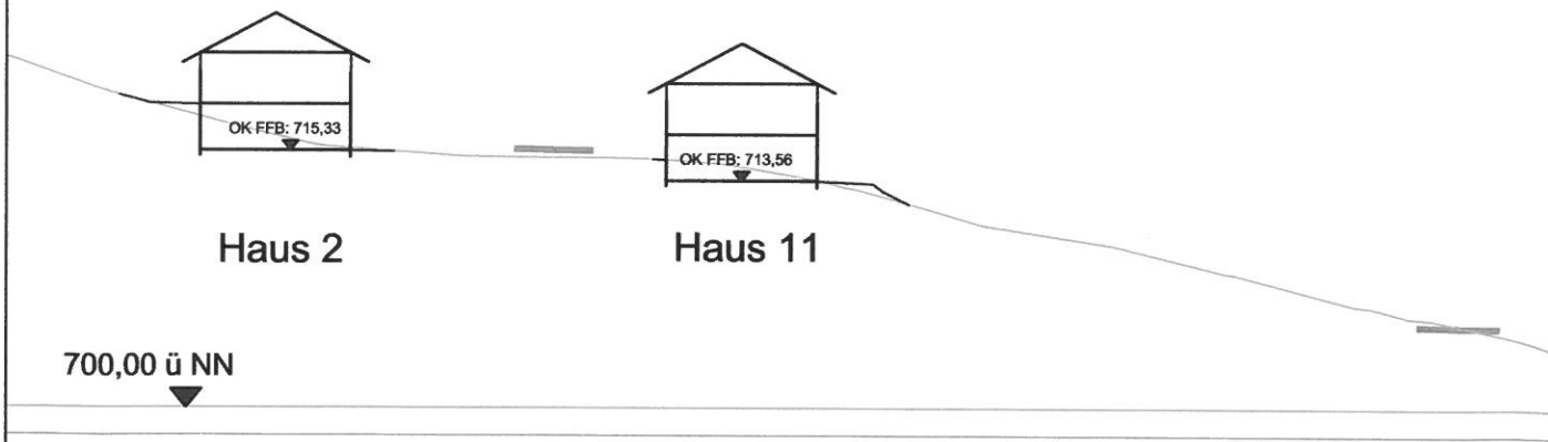
Schnitt 1 - 1; M 1 : 500
